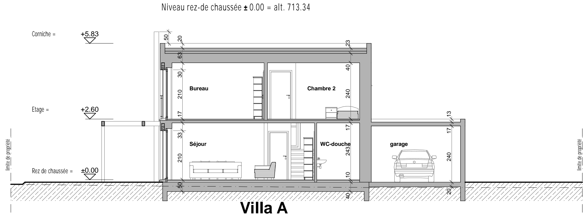
Coupe A-A
