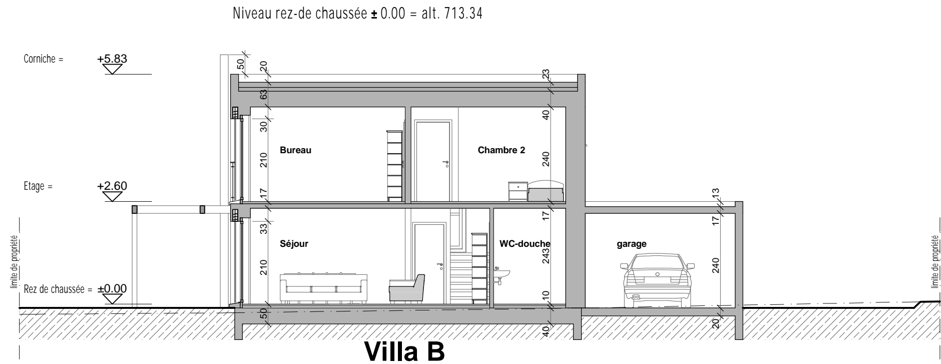
Coupe A-A
